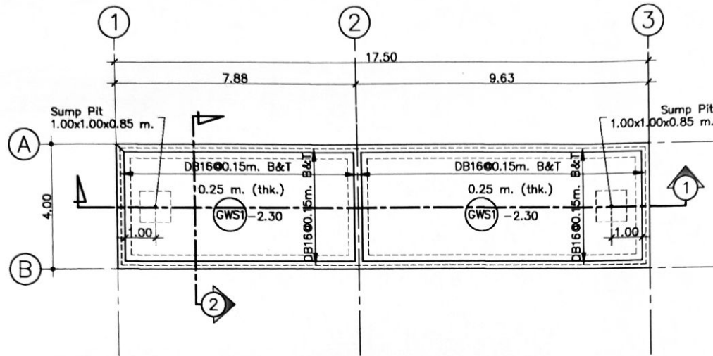
ระดับฐานราก
