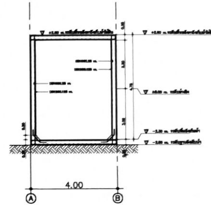
รูปตัด 2
